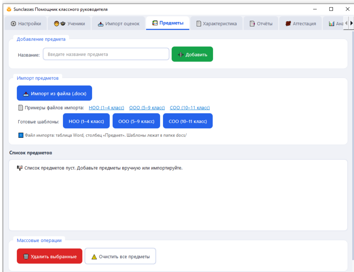
Рис.4 вкладка Предметы
